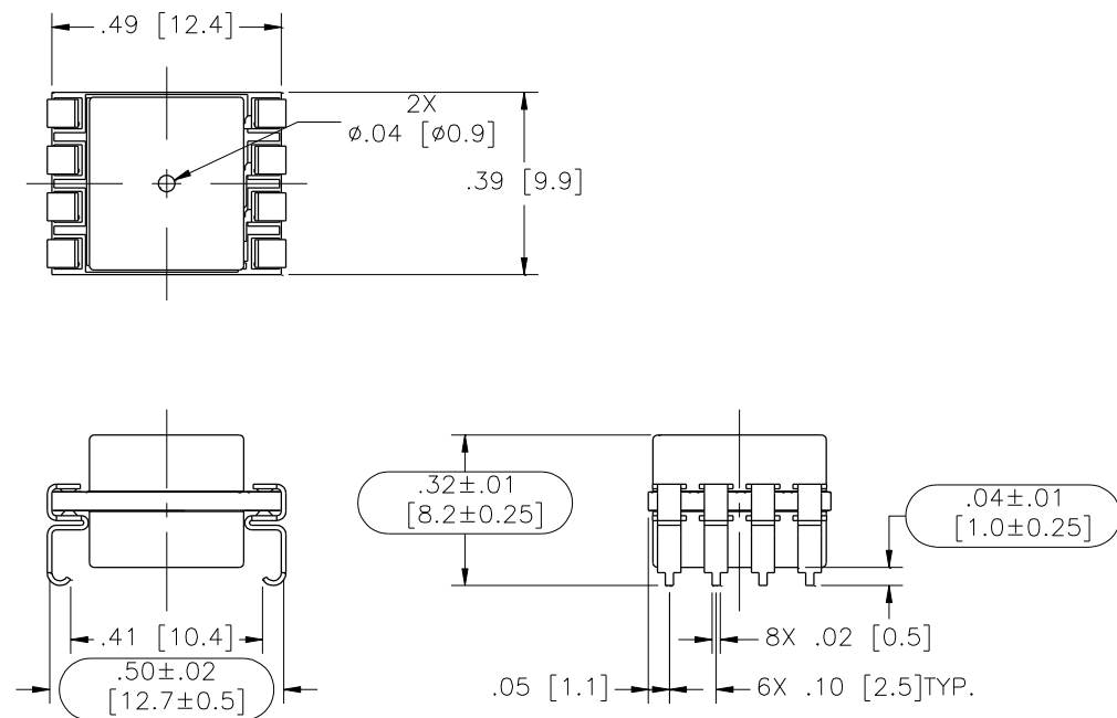
Model: MS4525DO-MMvoixxyS
