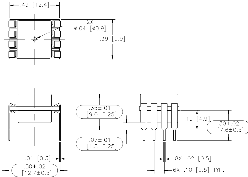
Model: MS4525DO-MMvoixxyP
